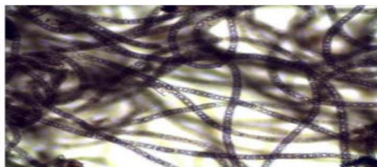
Слика 15. Microspora amoena (микроскопски изглед)
