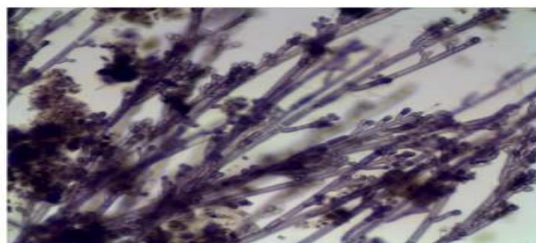
Слика 13. Audouinella chalybea (микроскопски изглед)
