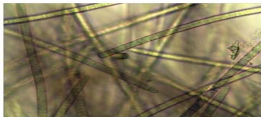
Слика 11. Phormidium favosum (микроскопски изглед)
